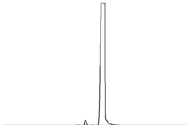
图 B.1 食品添加剂庚酸乙酯气相色谱图
