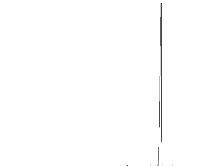
图 B.1 食品添加剂大茴香醛典型气相色谱图
