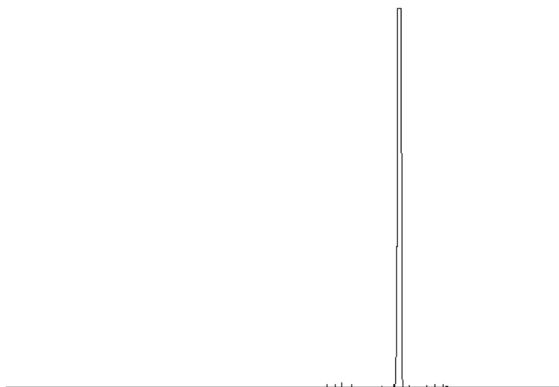
图 B.1 食品添加剂苯乙酸乙酯典型气相色谱图
