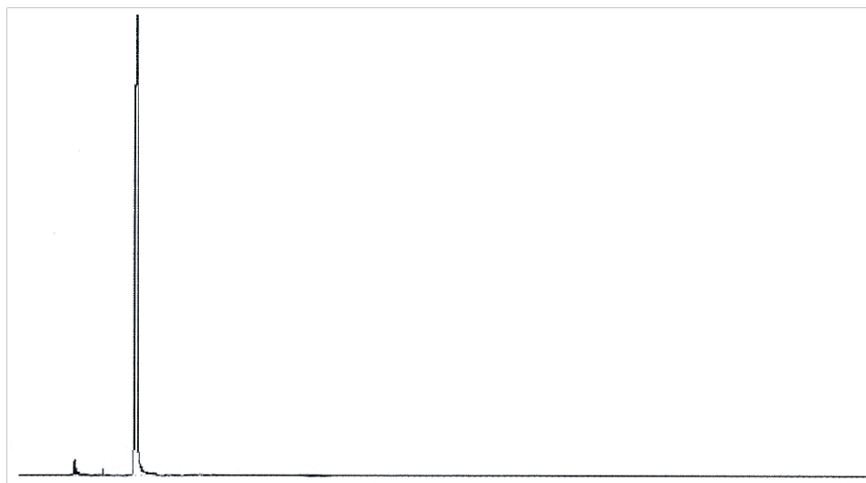
图 B.1 食品添加剂二甲基二硫醚气相色谱图
