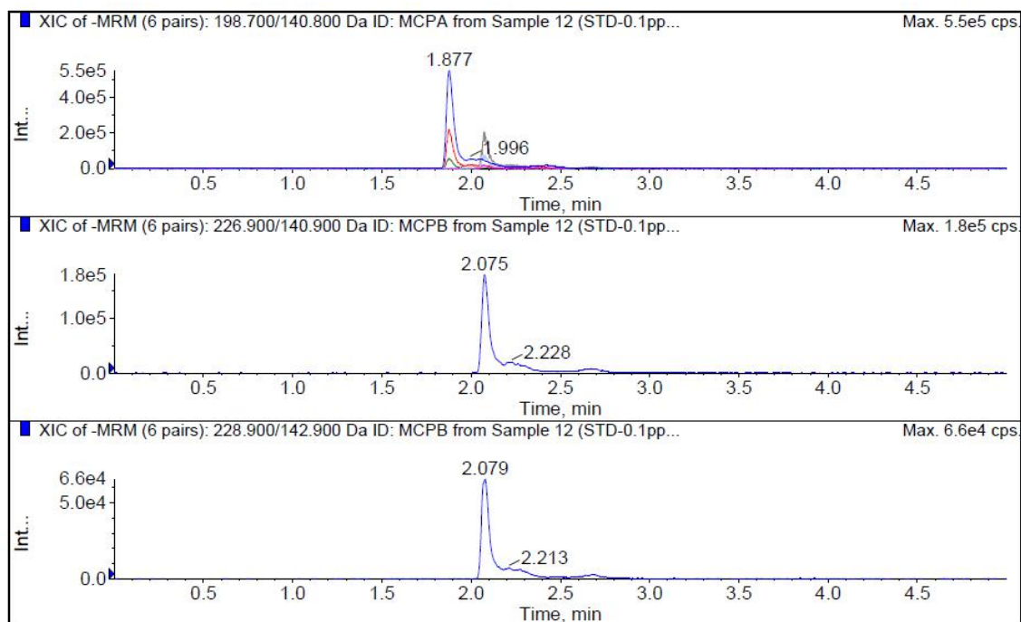
图 B.2 MCPB 标准品 LC-MS/MS MRM 图
