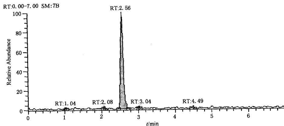
图 A.1 氨本砷标准溶液特征离子质量色谱图(0.5 µg/L)
