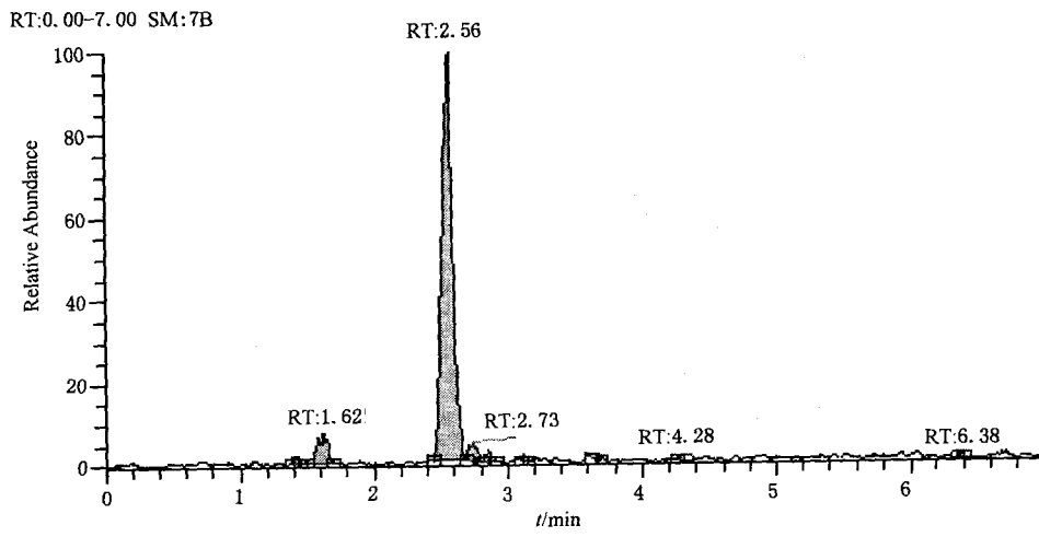
图 A.3 猪肝组织空白添加氨本砒试样特征离子质量色谱图(0.5 \mu\text{g}/\text{kg} )
