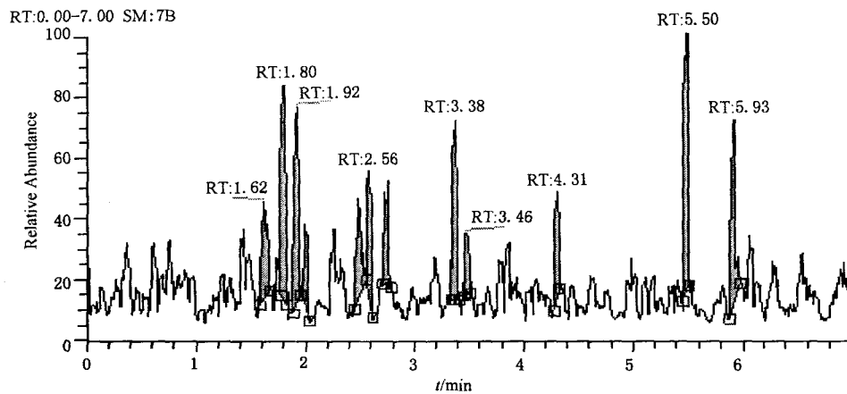
图 A.2 猪肝脏组织空白试样特征离子质量色谱图
